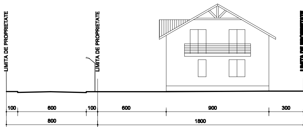
SECTIUNE TRANSVERSALA sc. 1: 100
